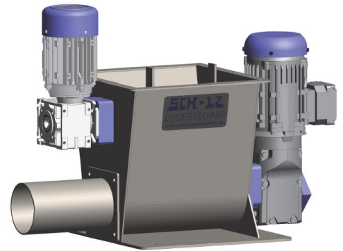
SOLO mit horizontalem Rohr mit Sonderausstattung Rührwerk
