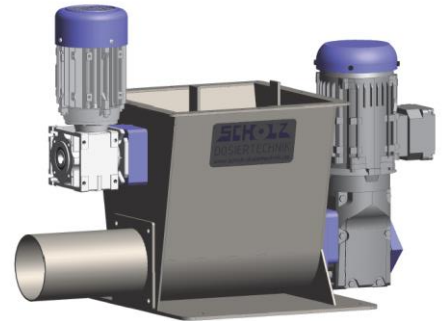
SOLO mit horizontalem Rohr mit Sonderausstattung Rührwerk
